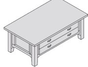
Konferenční stůl, 4 zásuvky š x v x h (mm): 1300x500x750
